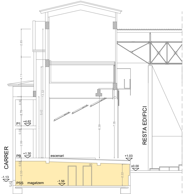
SECCIÓ LONGITUDINAL A-A
