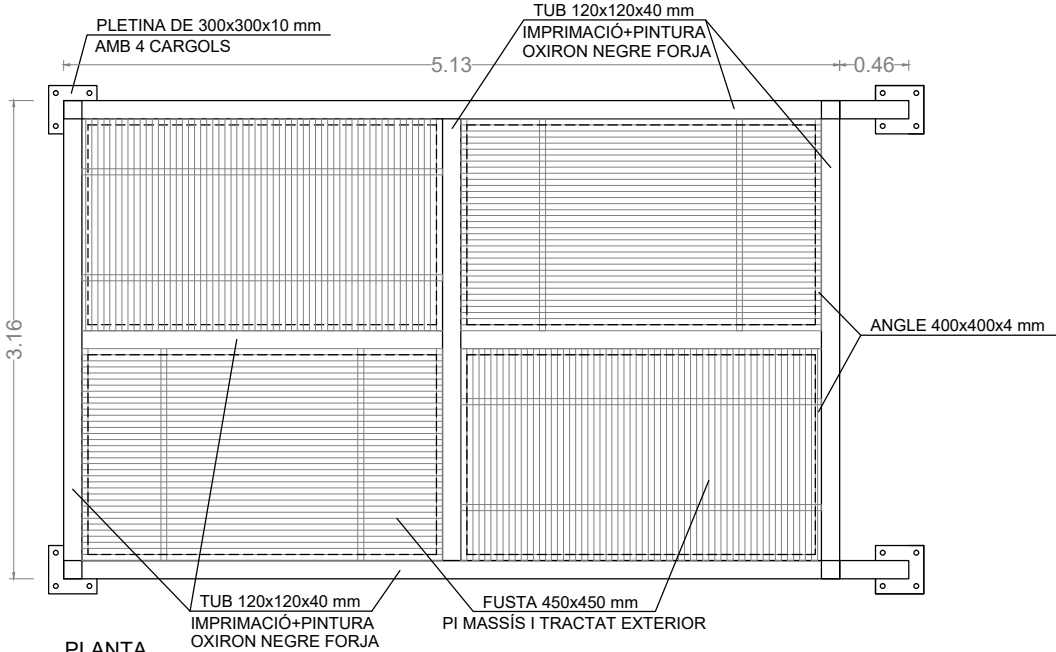
PLANTA
