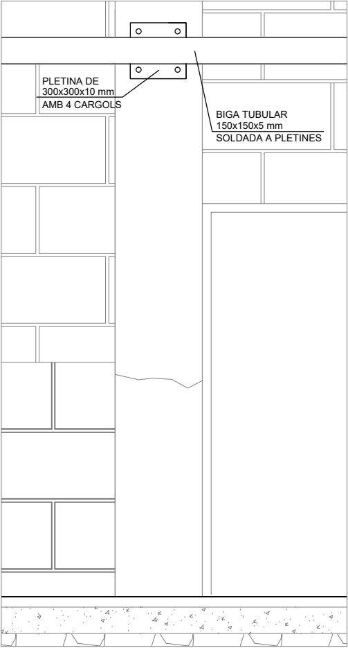
DETALL C (ALÇAT)
