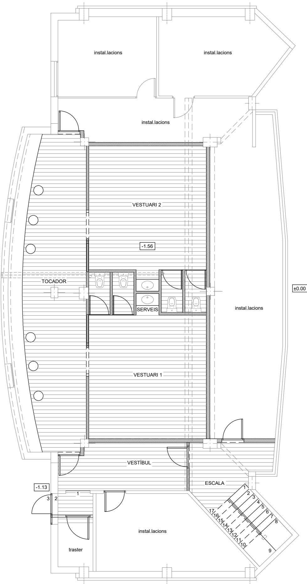
PLANTA SEMISOTERRANI
