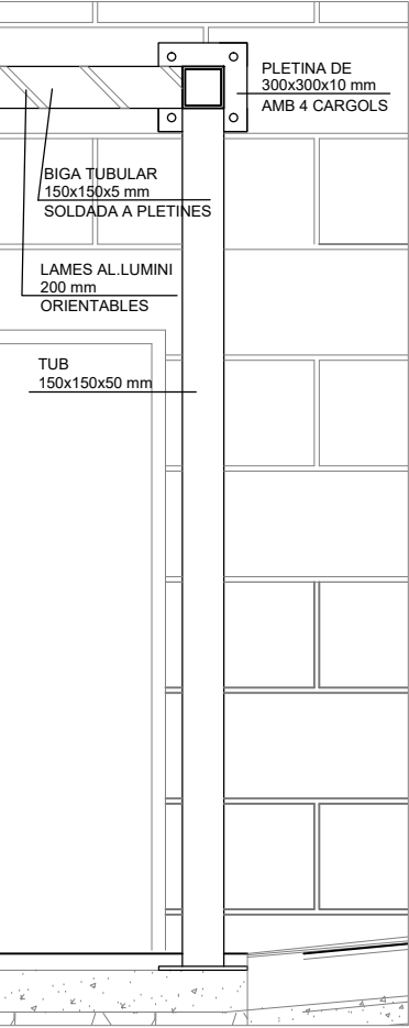
DETALL B (ALÇAT)
