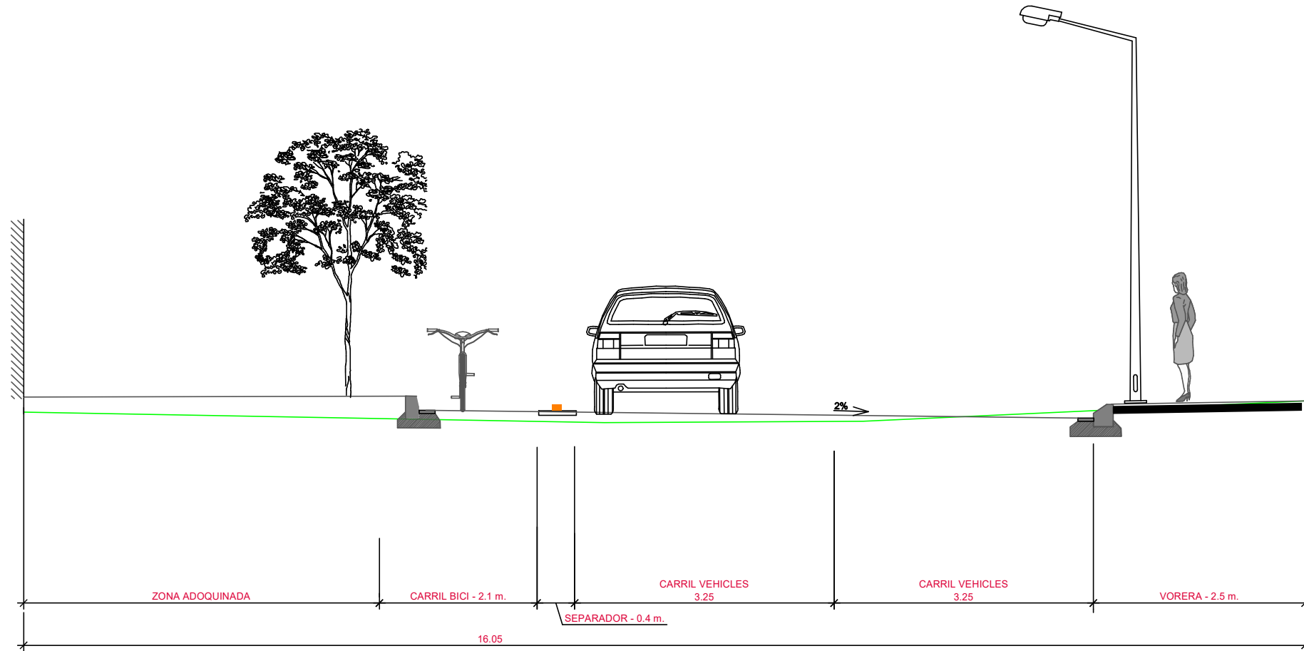
SECCIÓ C-C' TRAM INTERMIG - ZONA ADOQUINADA LATERAL
