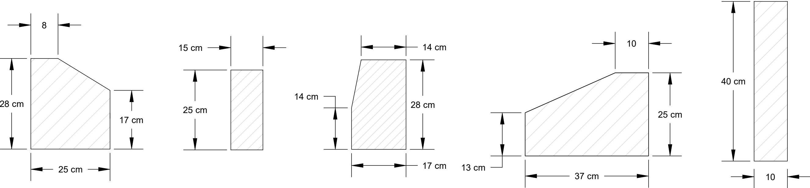
VORADA DE FORMIGO PREFABRICAT REMONTABLE (L=50cm)
