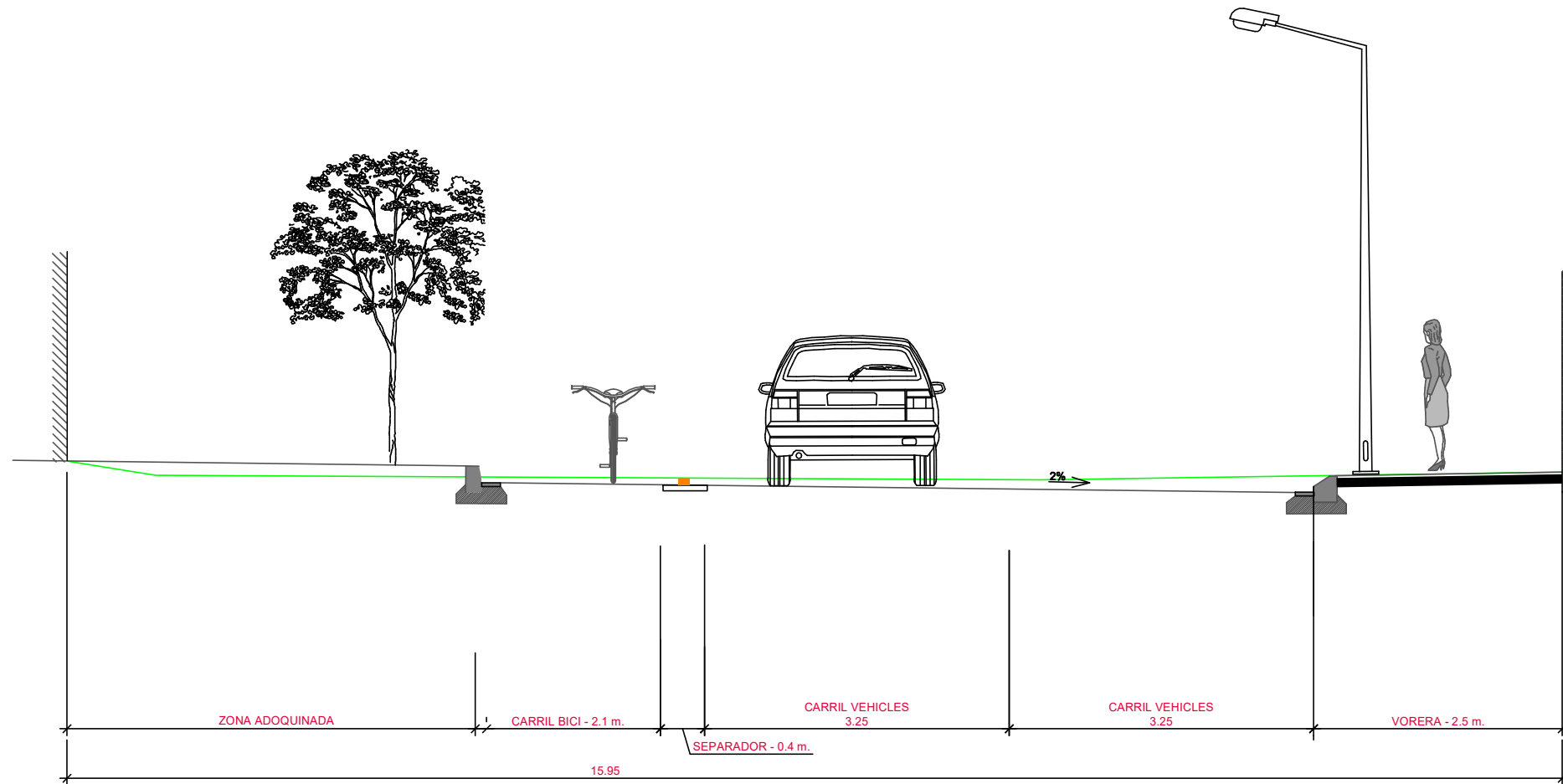
SECCIÓ A-A' TRAM INICIAL - ZONA ADOQUINADA LATERAL
