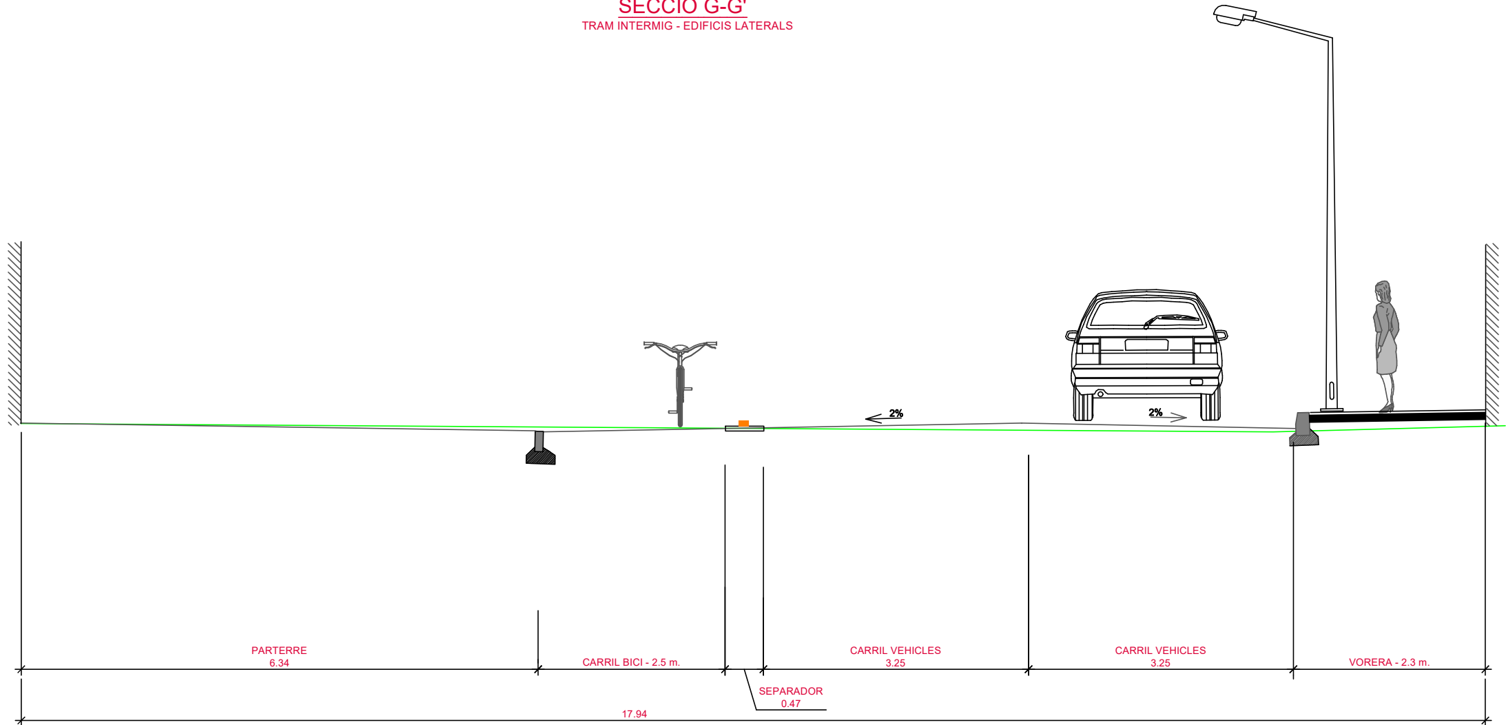
SECCIÓ F-F' TRAM INTERMIG - EDIFICIS LATERALS
