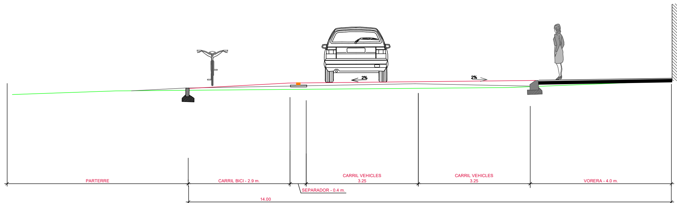
SECCIÓ D-D' TRAM INTERMIG-ACCES IMMOBLES
