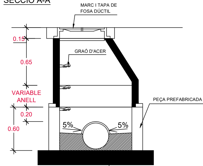
SECCIÓ A-A
