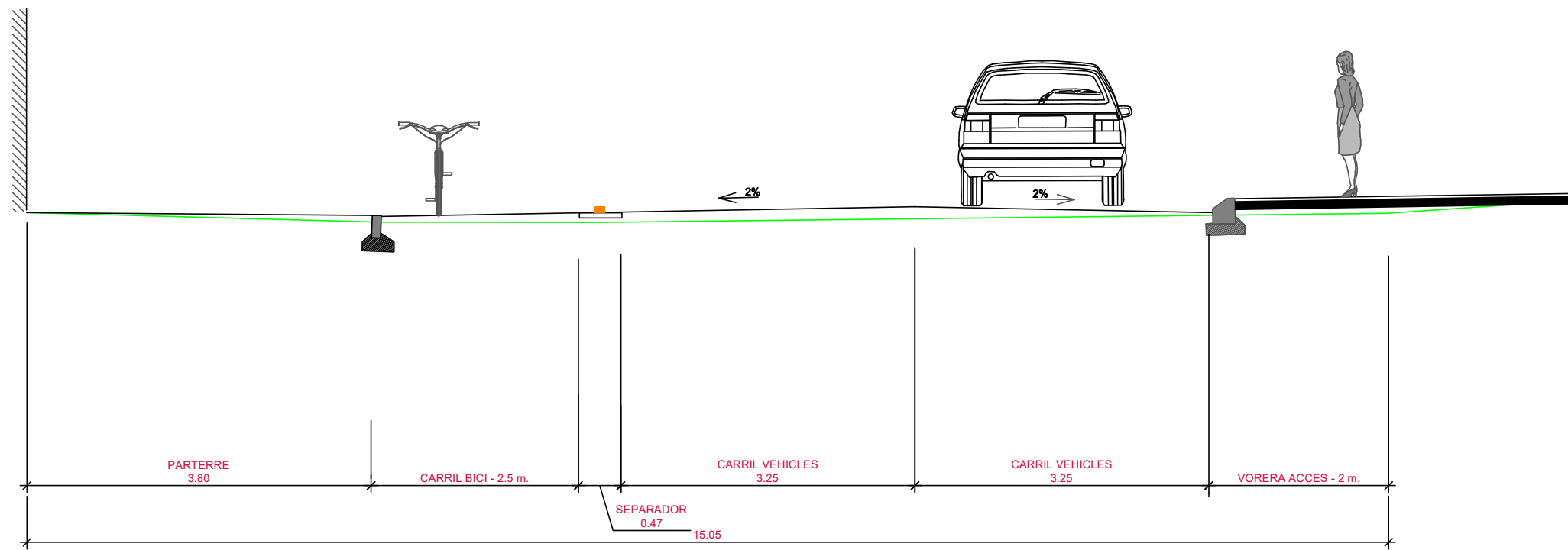
SECCIÓ I-I' TRAM FINAL - ACCES IMMOBLE
