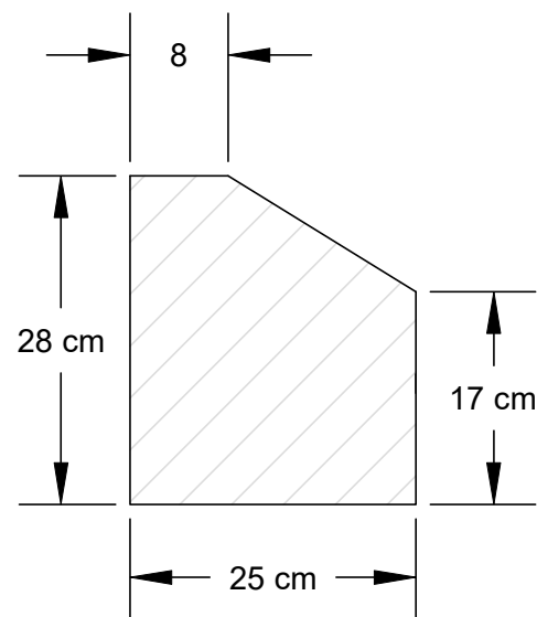
VORADA DE FORMIGO PREFABRICAT REMONTABLE (L=50cm)
