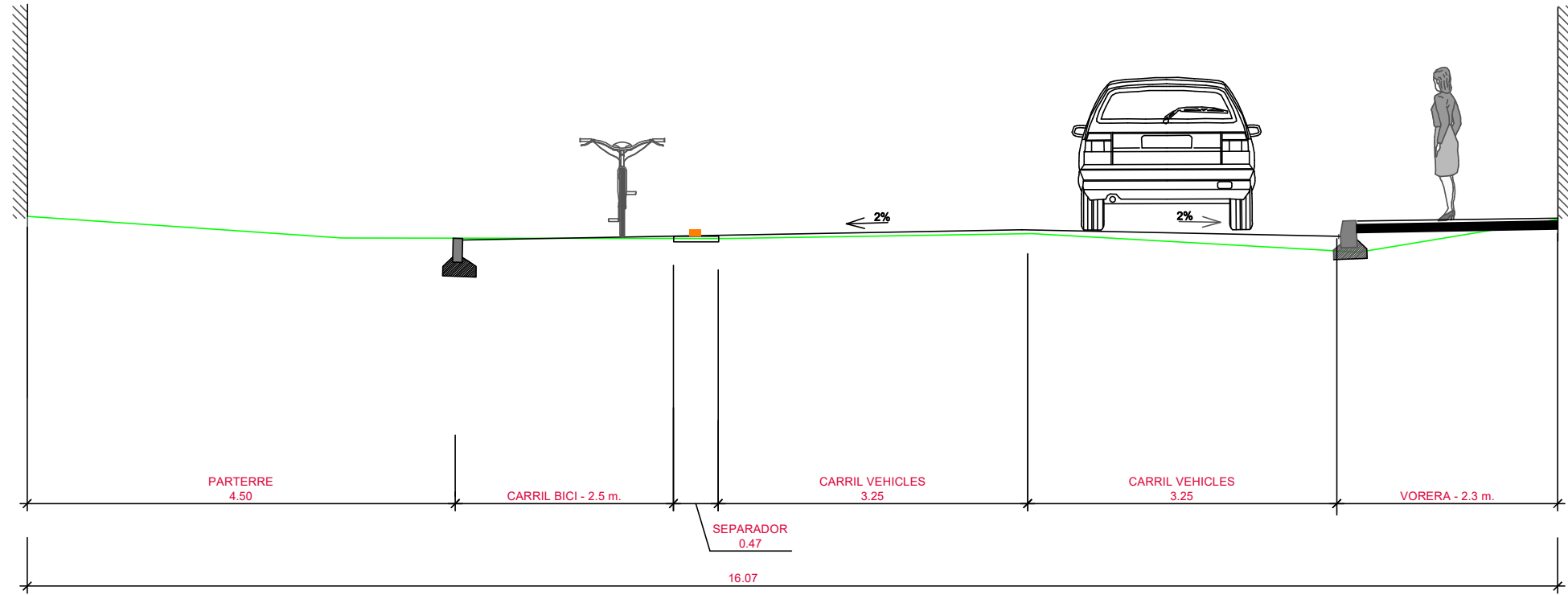
SECCIÓ G-G' TRAM INTERMIG - EDIFICIS LATERALS
