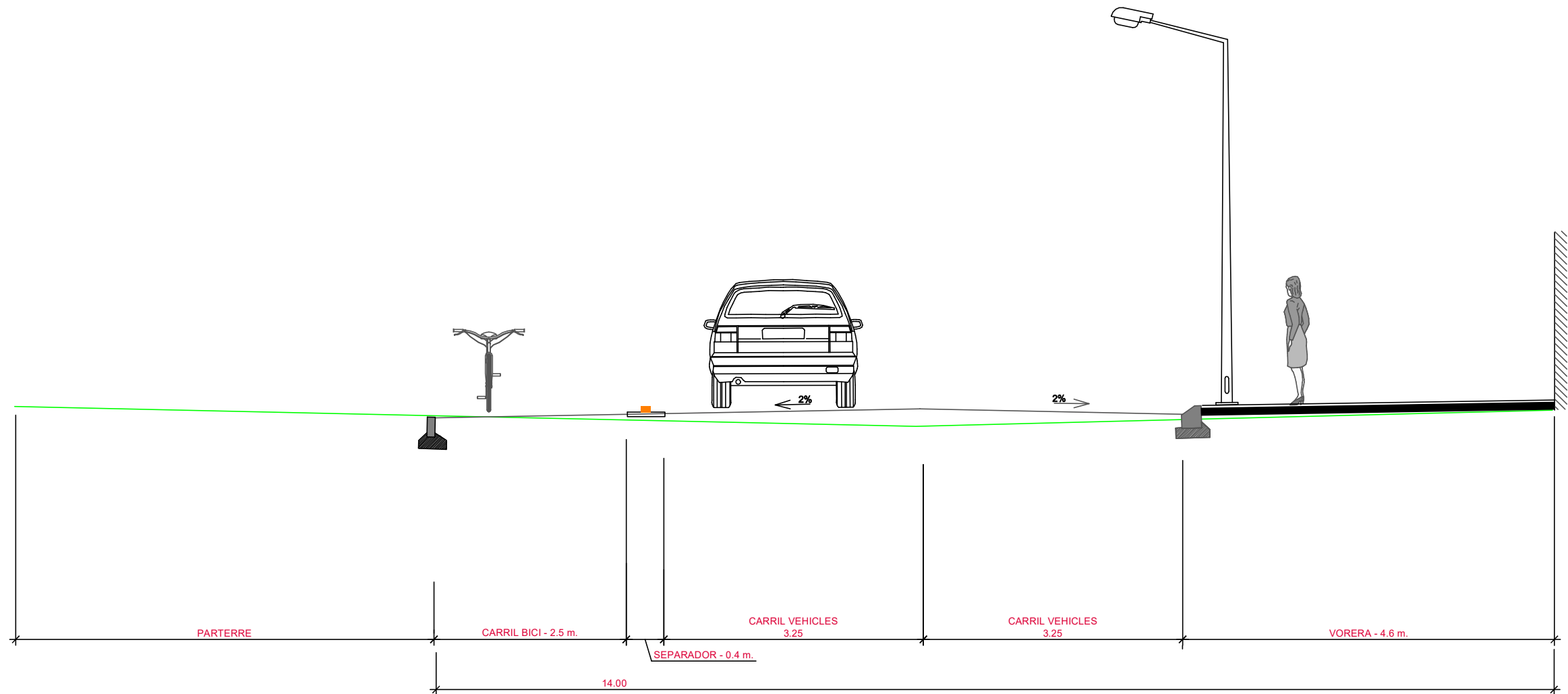
SECCIÓ E-E' TRAM INTERMIG-ACCES IMMOBLES
