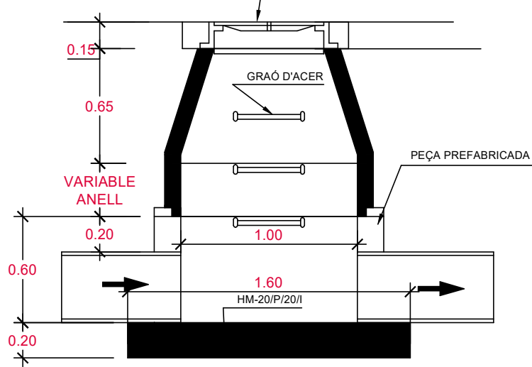
SECCIÓ B-B
