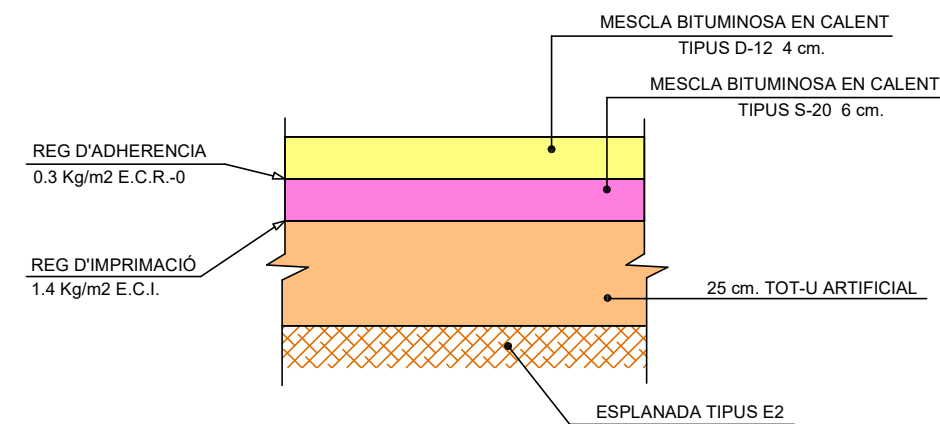
PAVIMENT ASFÀLTIC. ESCALA S/E
